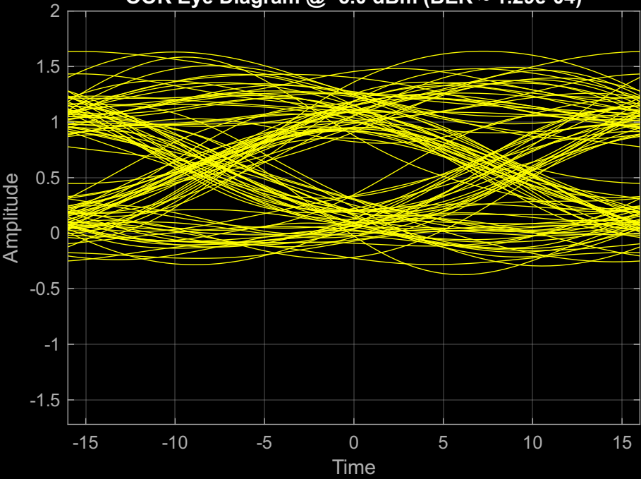
OOK Eye Diagram @ -5.0 dBm (BER \approx 1.29\text{e-}04 )
